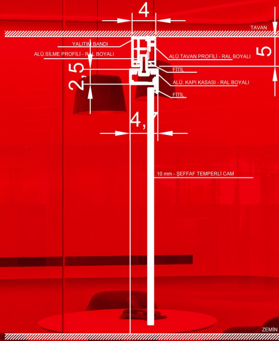
KLASSE MODÜLER BÖLME DUVAR (TEK CAMLI CAM CAMA BİRLEŞİMLİ)
